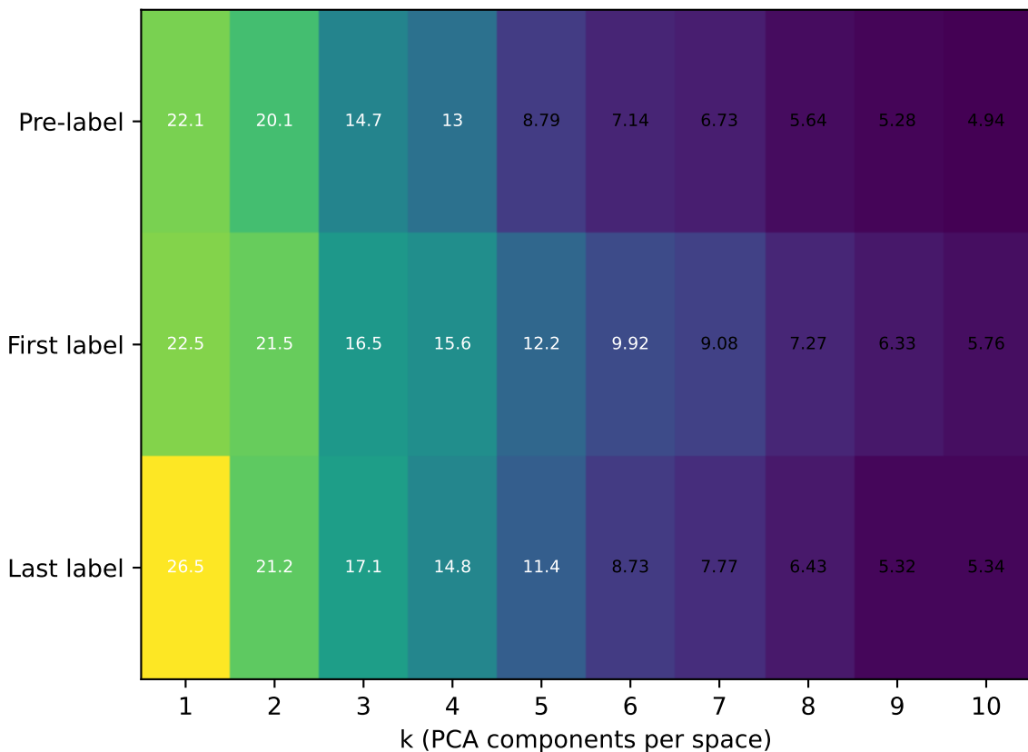
Train-task MSE
