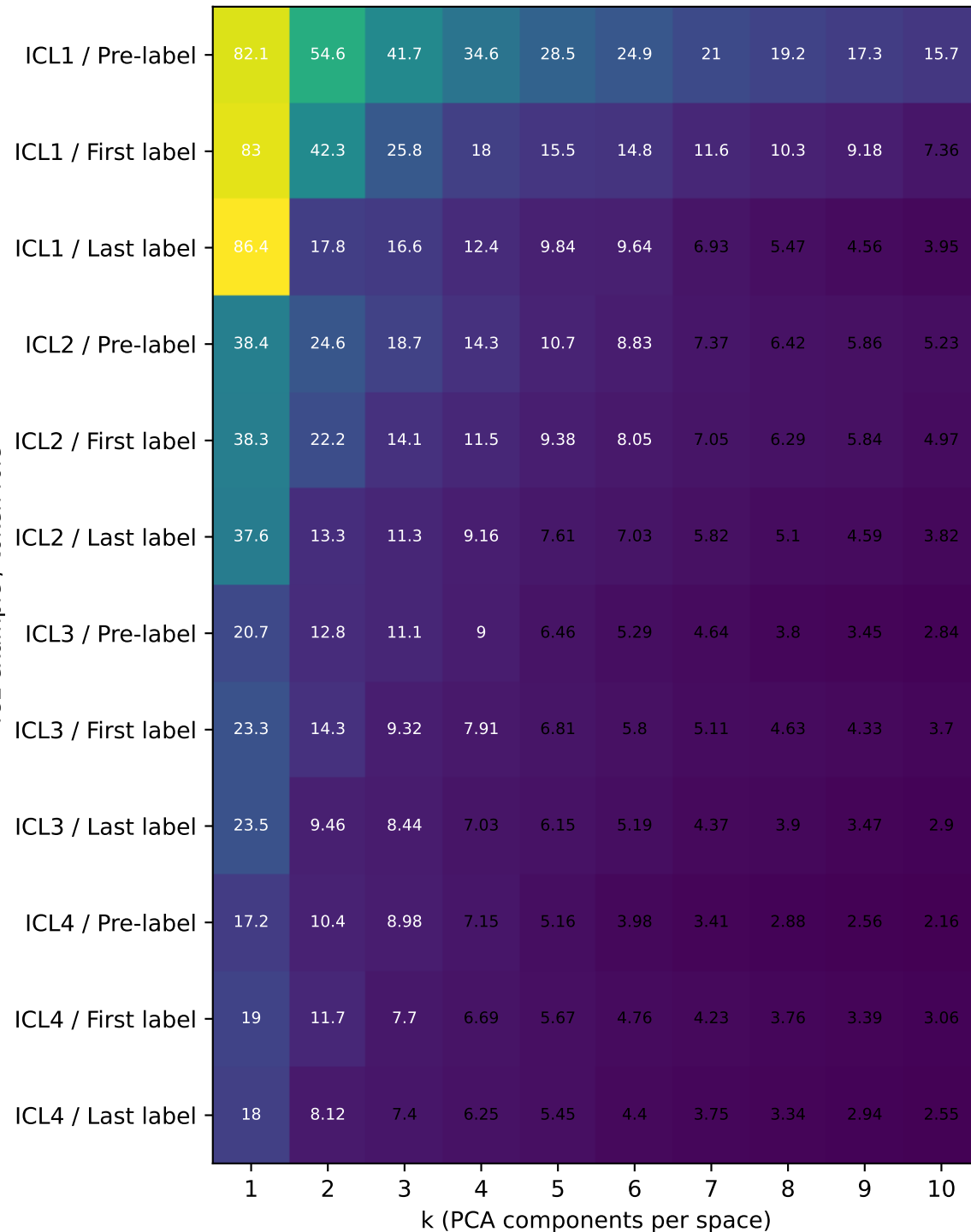
Train-task MSE
