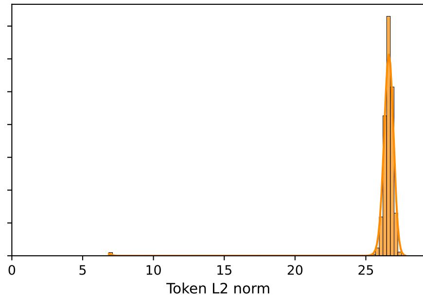
PNG DeiT-B
