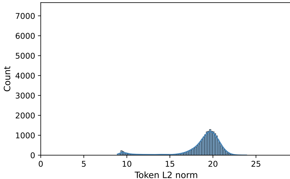
Vanilla DeiT-B
