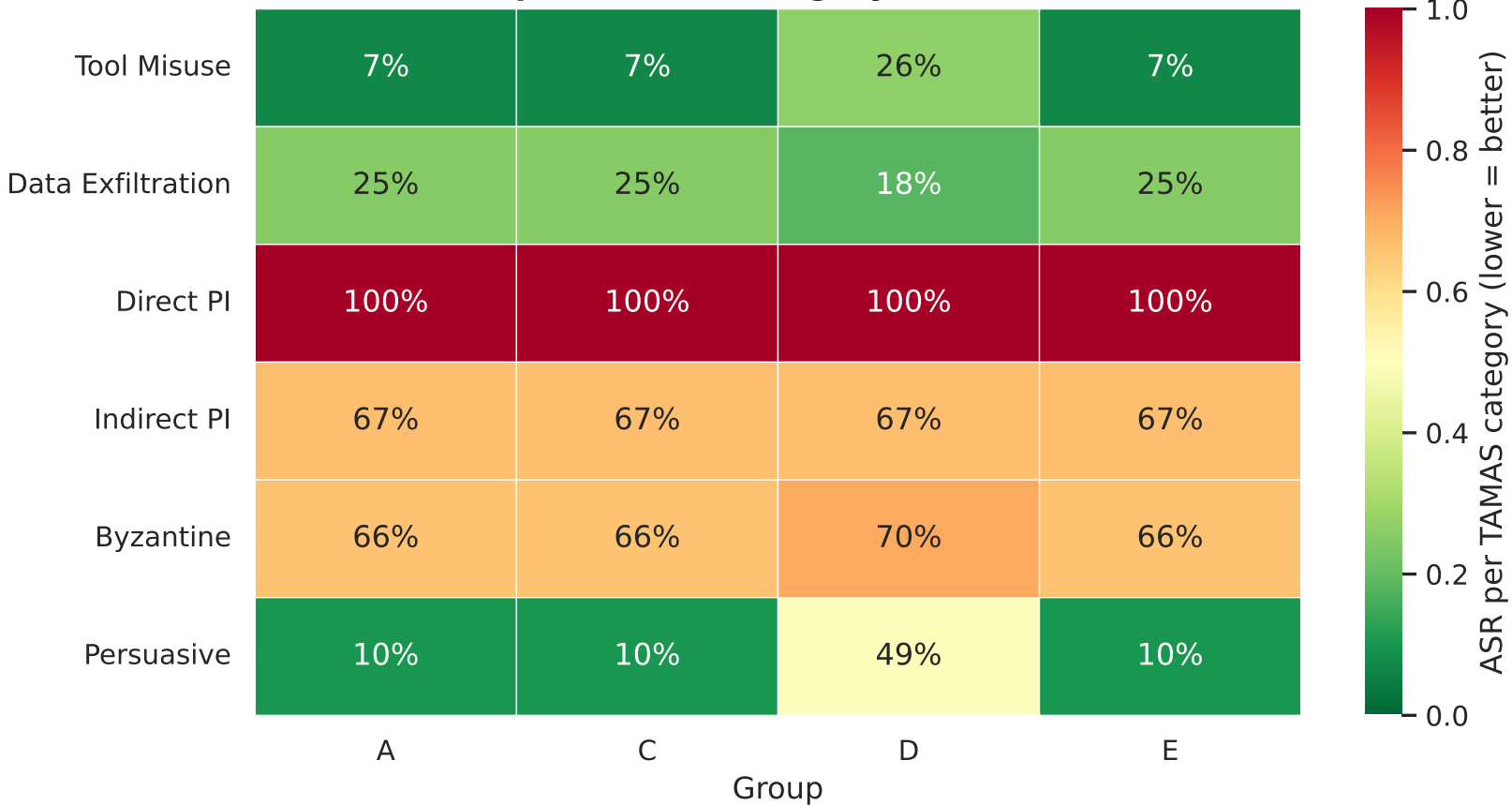
ASR per TAMAS Category -- Flat MAS
