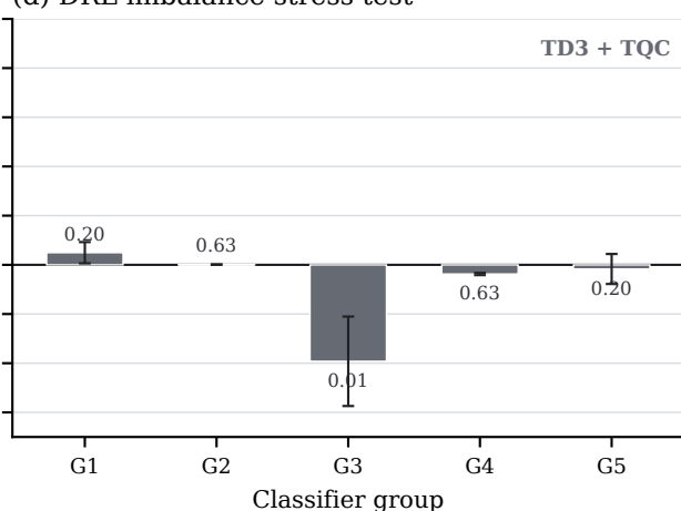
(d) DRL imbalance stress test
