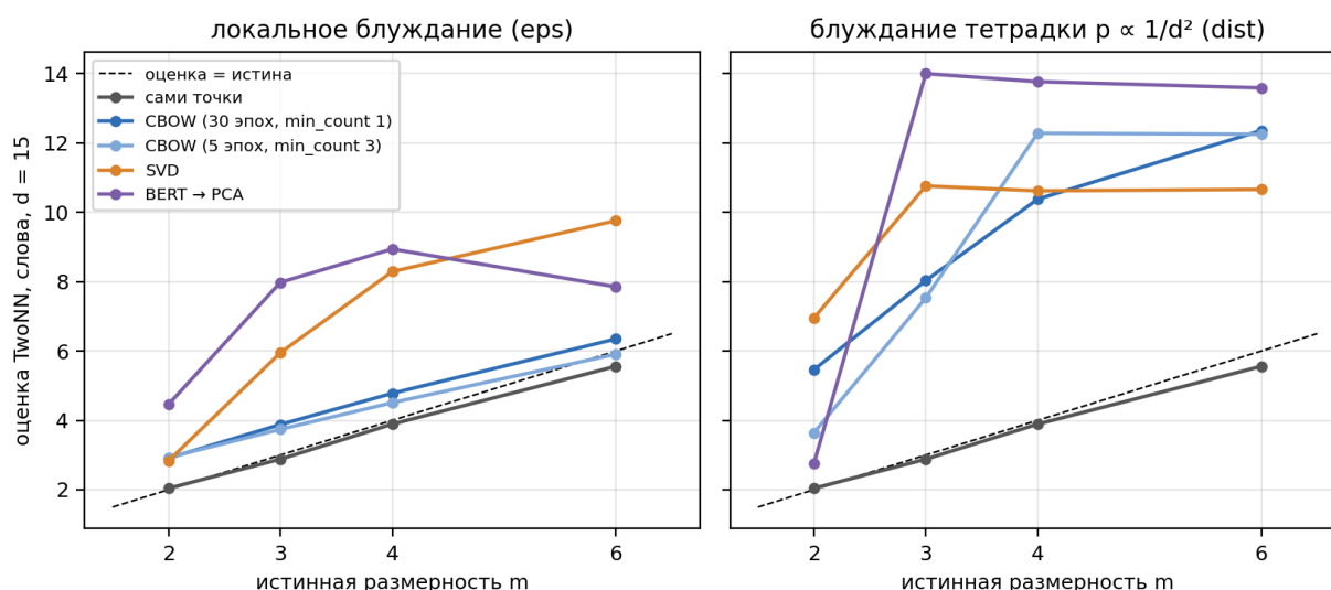
Рис. 1. TwoNN по словам при d = 15 против истинной m . Слева (eps): оба CBOV идут вдоль диагонали чуть выше неё; SVD и BERT → PCA сильно завышают, BERT не различает m = 3-6 . Справа (dist, отрицательный контроль): текст почти случаен, все эмбединги далеко от истины.
