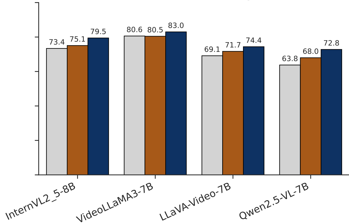
MLVU (Subset Average)
