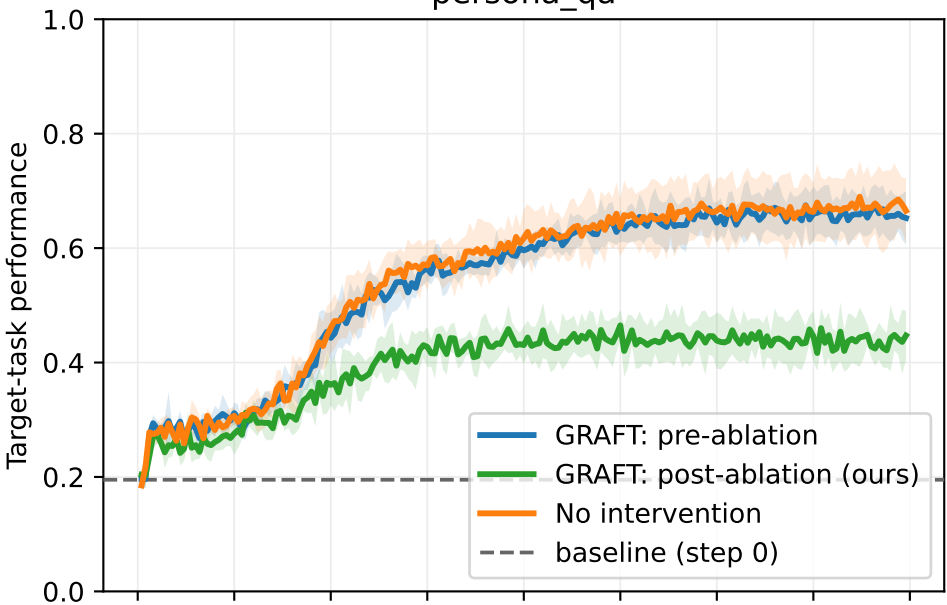
persona_qa
