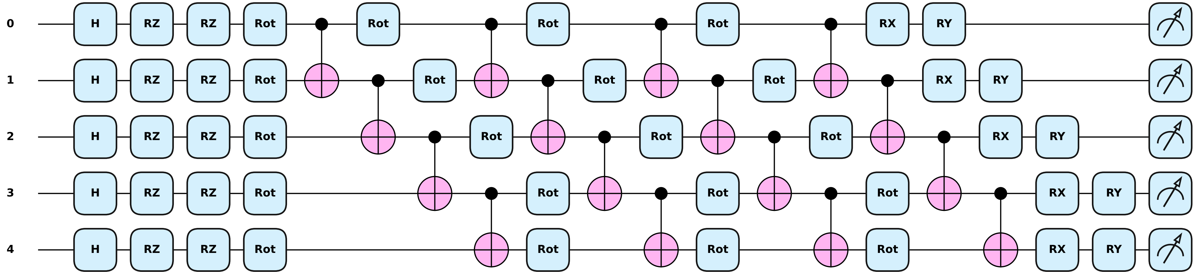
V3 - 5 qubits x 4 layers x linear topology - 75 parameters
