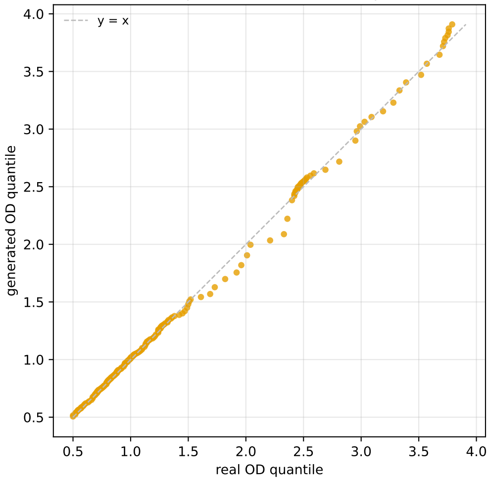
Q-Q plot — Quantum V3 (75p)
