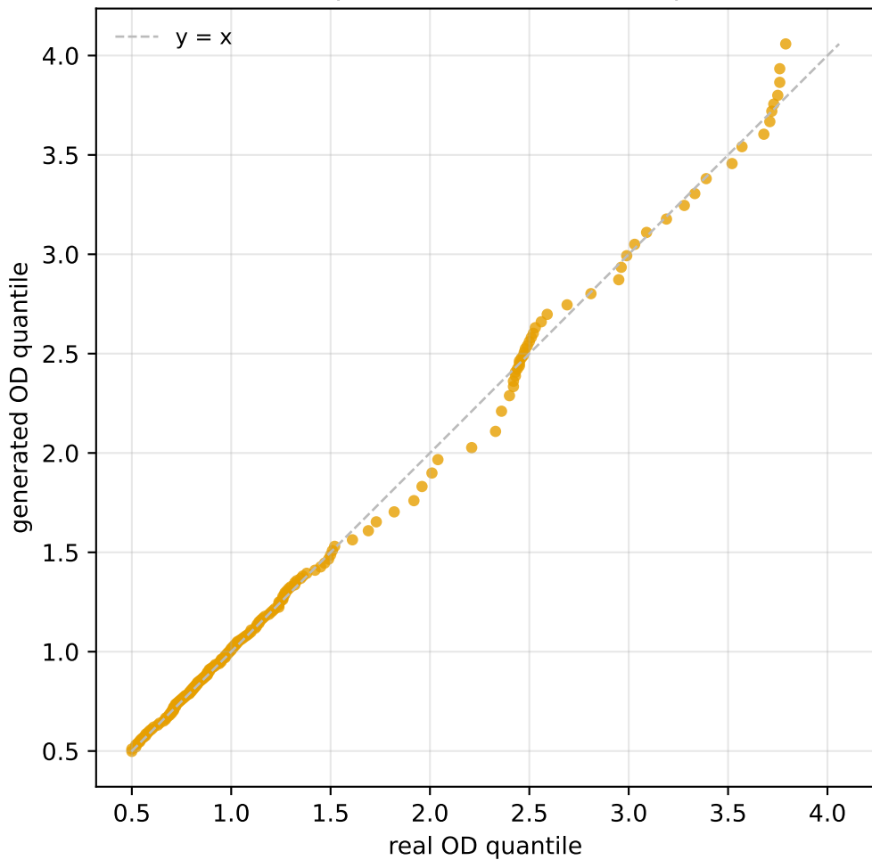
Q-Q plot — Quantum V3 (75p)
