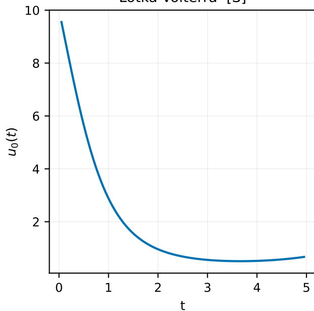
Lotka-Volterra [S]
