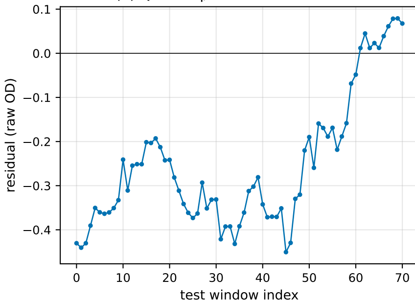
(d) QLNN 4q/3L — residual vs time
