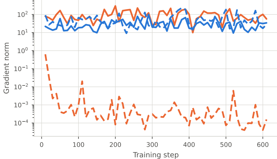
(d) Gradient norm
