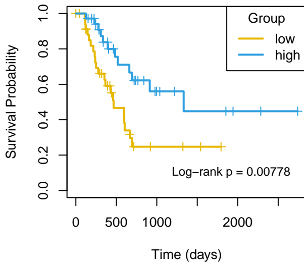
DSS mir-502
