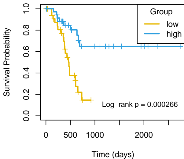
DSS mir-98
