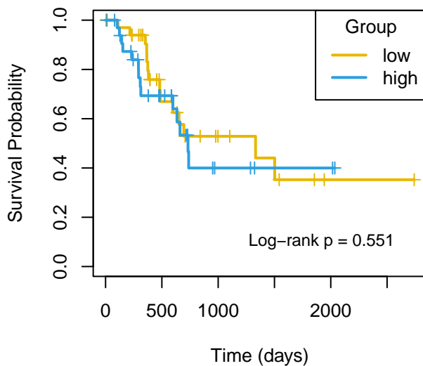
DSS mir-27a
