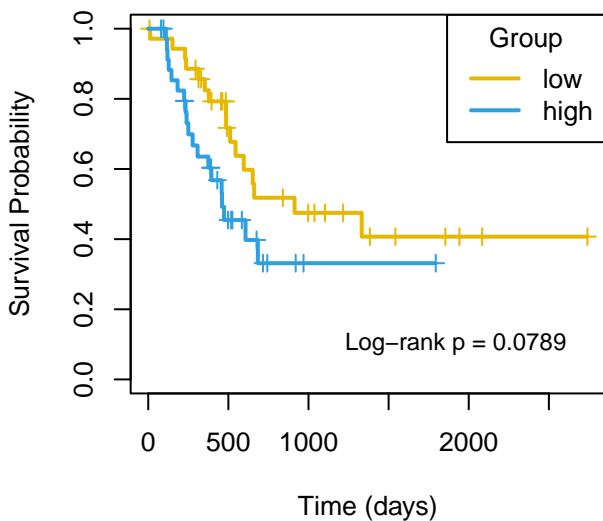
OS mir-21
