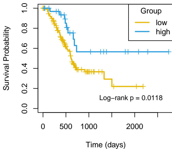
DSS mir-3609
