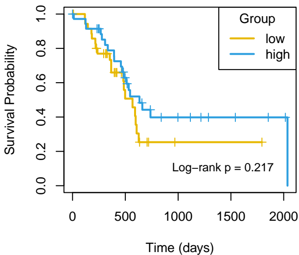
OS mir-200b
