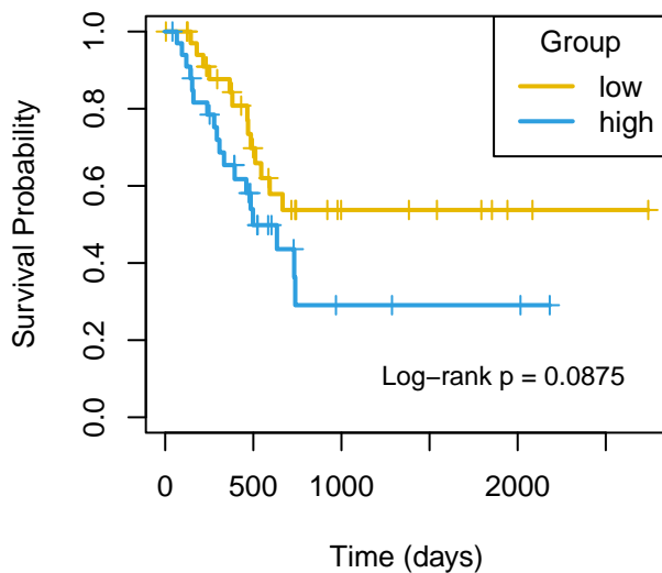
DSS mir-31
