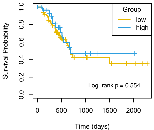
DSS mir-320c-2
