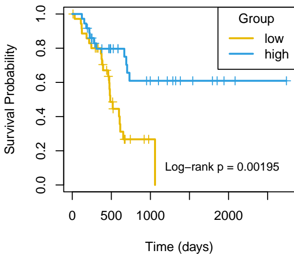
OS mir-301a
