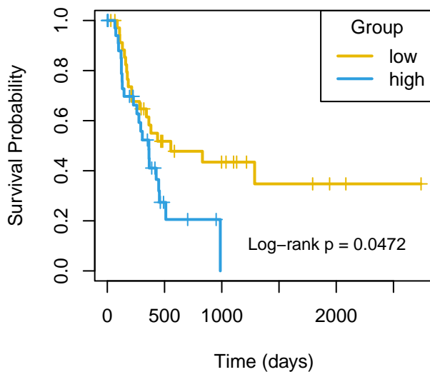
PFI mir-503
