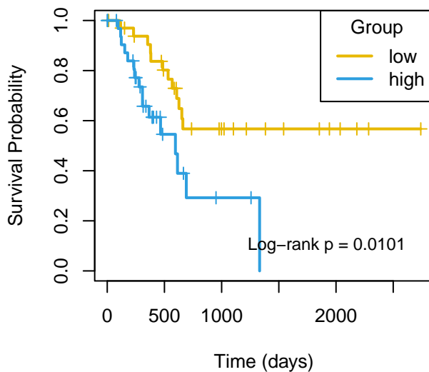
DSS mir-3922
