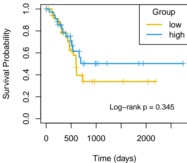
DSS mir-660
