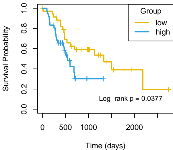
OS mir-205
