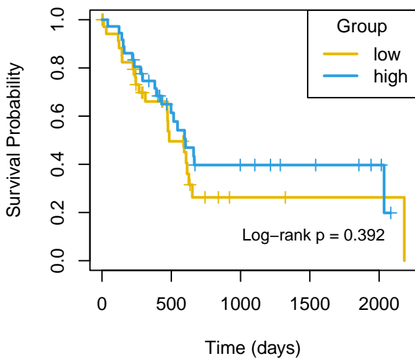
OS mir-1343
