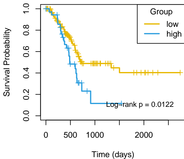
DSS mir-3138
