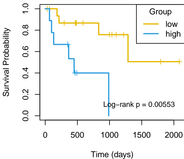
DFI mir-503
