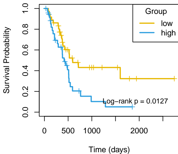
PFI mir-509-1
