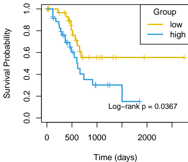
DSS mir-193a
