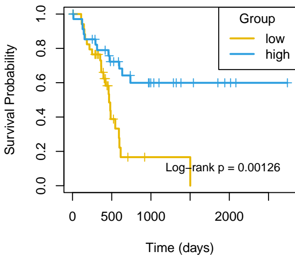
OS mir-29b-1
