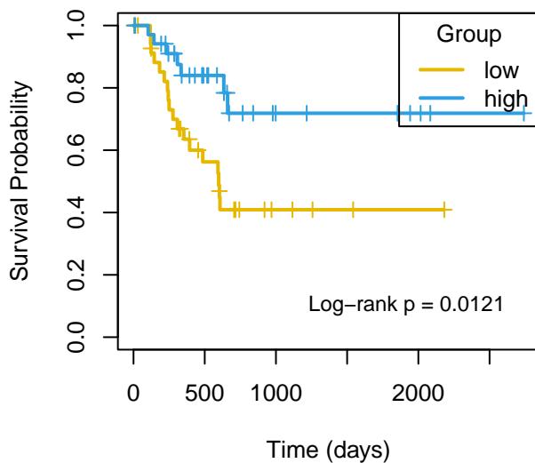
DSS mir-500b
