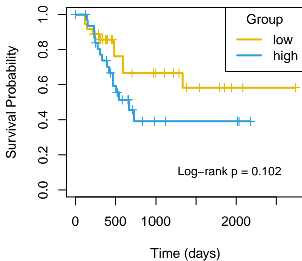
DSS mir-203b
