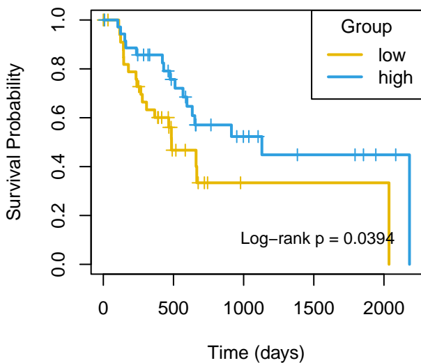
OS mir-885
