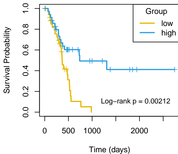
PFI mir-3613
