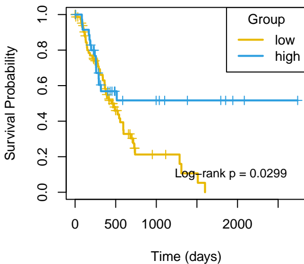
PFI mir-488
