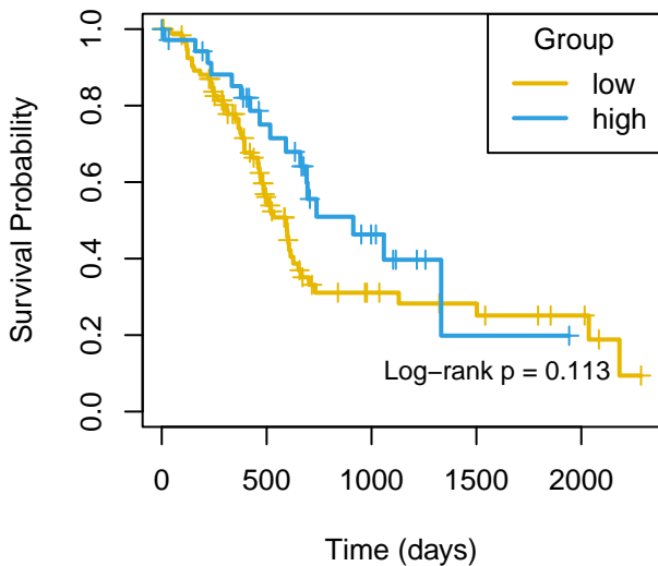
OS mir-5003
