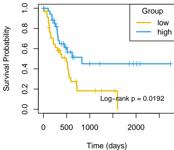
PFI mir-500b
