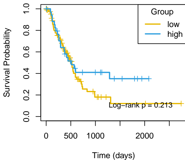
PFI mir-544a
