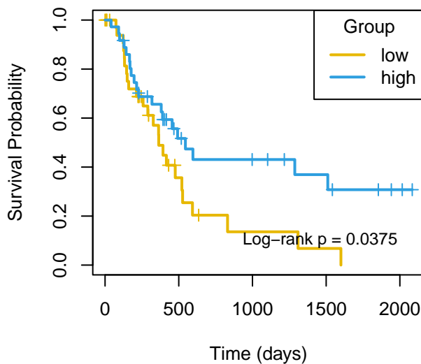
PFI mir-1343
