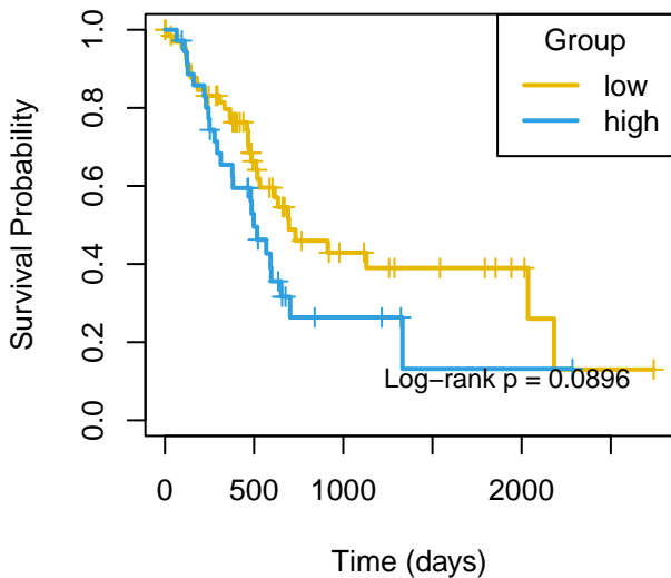
OS mir-548o-2
