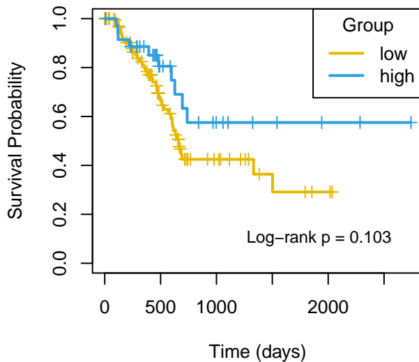
DSS mir-5680
