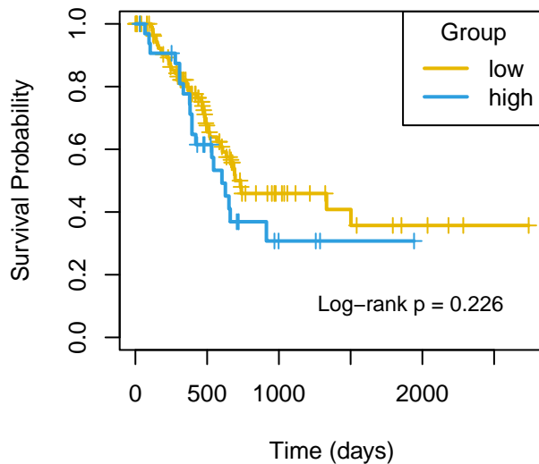
DSS mir-4727
