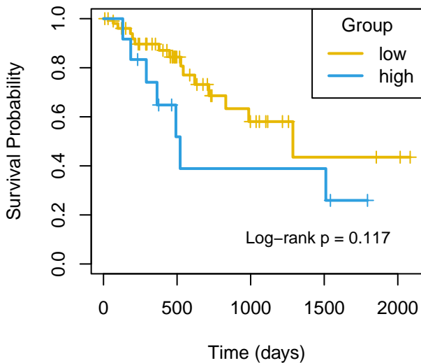
DFI mir-548n
