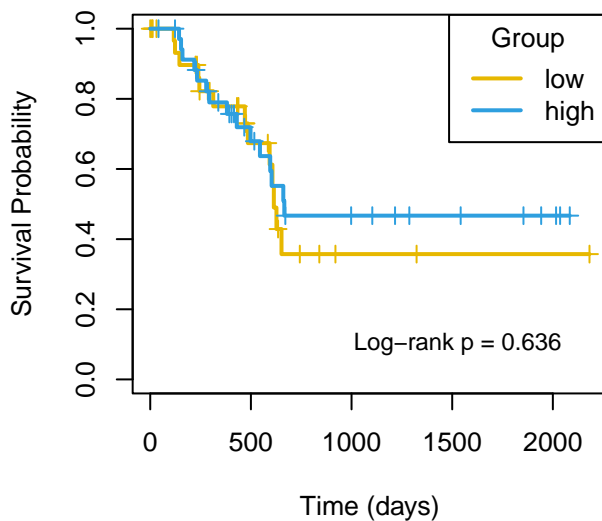
DSS mir-1343
