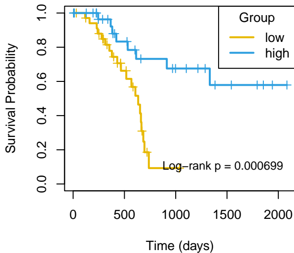
DSS mir-5010
