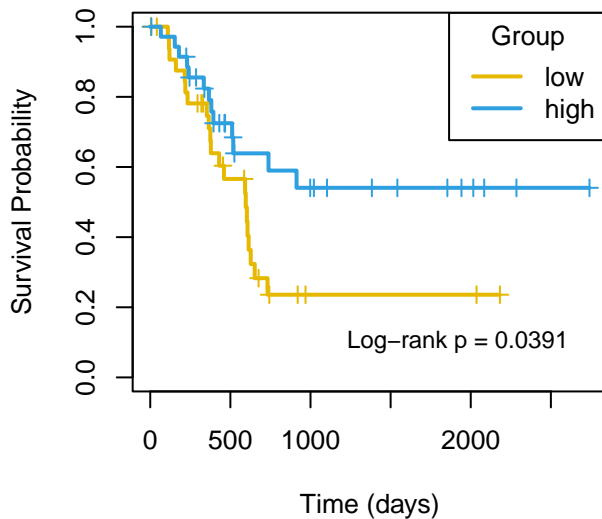
DSS mir-361
