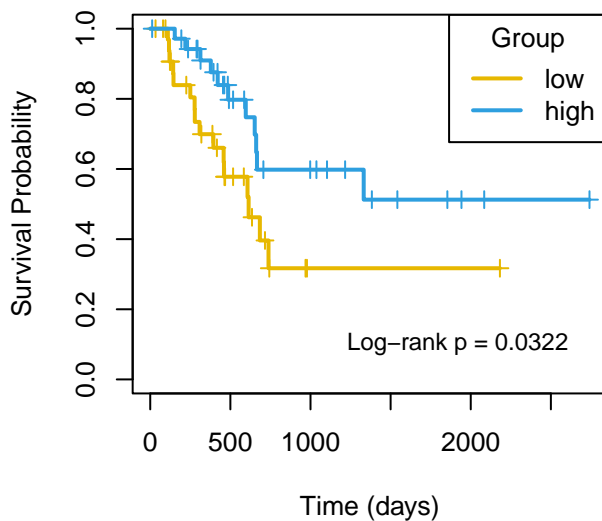
DSS mir-375
