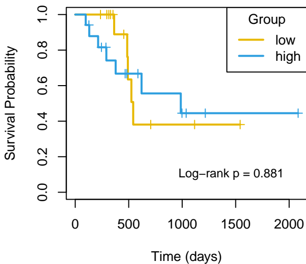
DFI mir-19b-1
