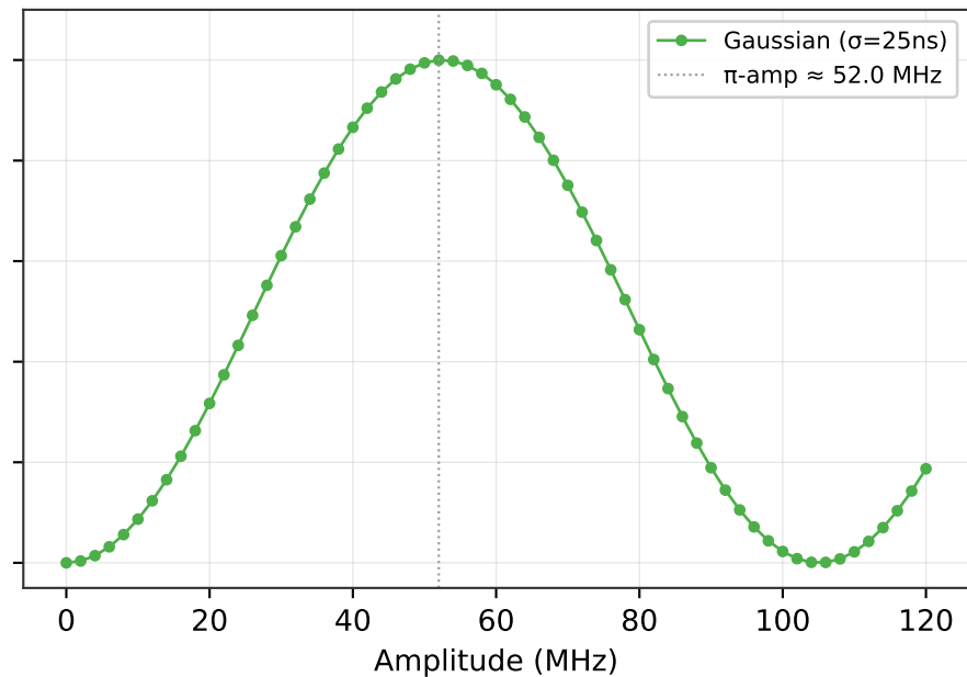
Gaussian Pulse ( \sigma=25 ns, T=100 ns)
