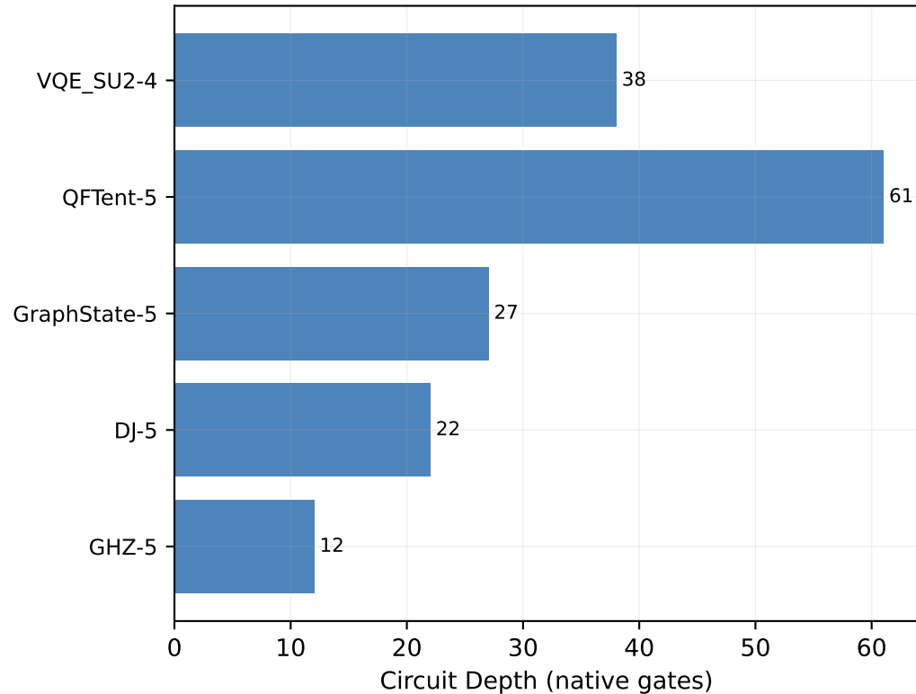
Pre-Transpile Depth
