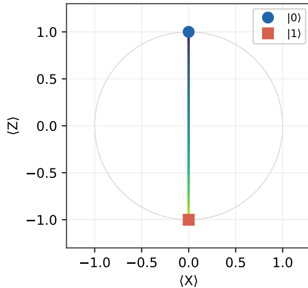
Bloch XZ ( \pi -pulse)
