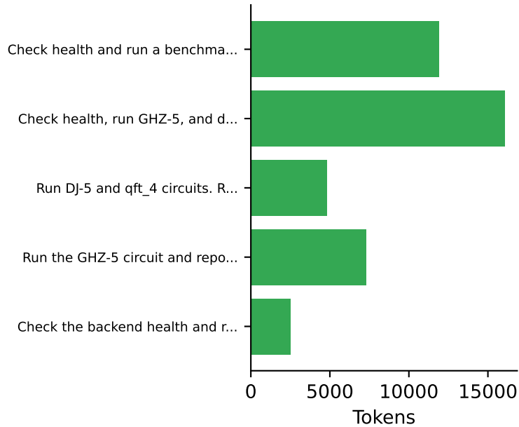
Token Usage per Session
