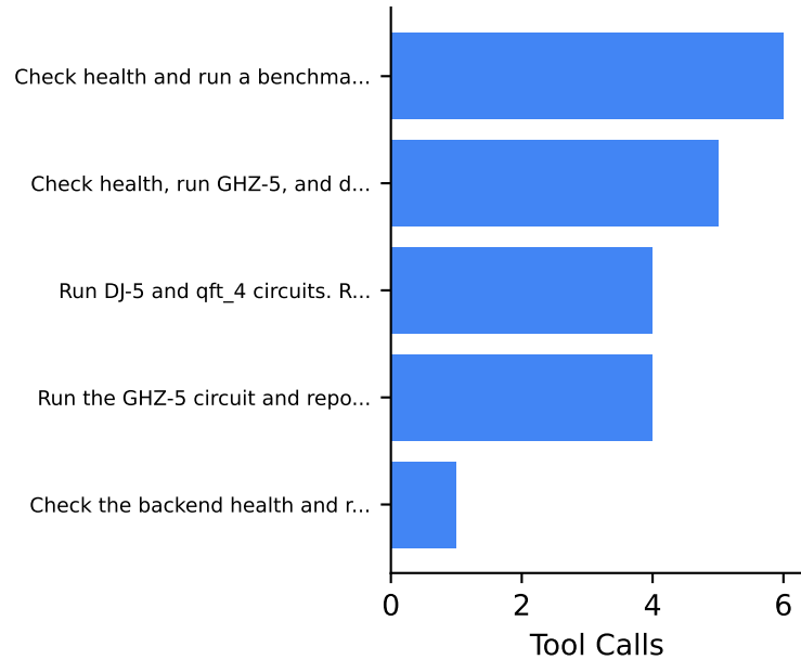
Tool Calls per Session
