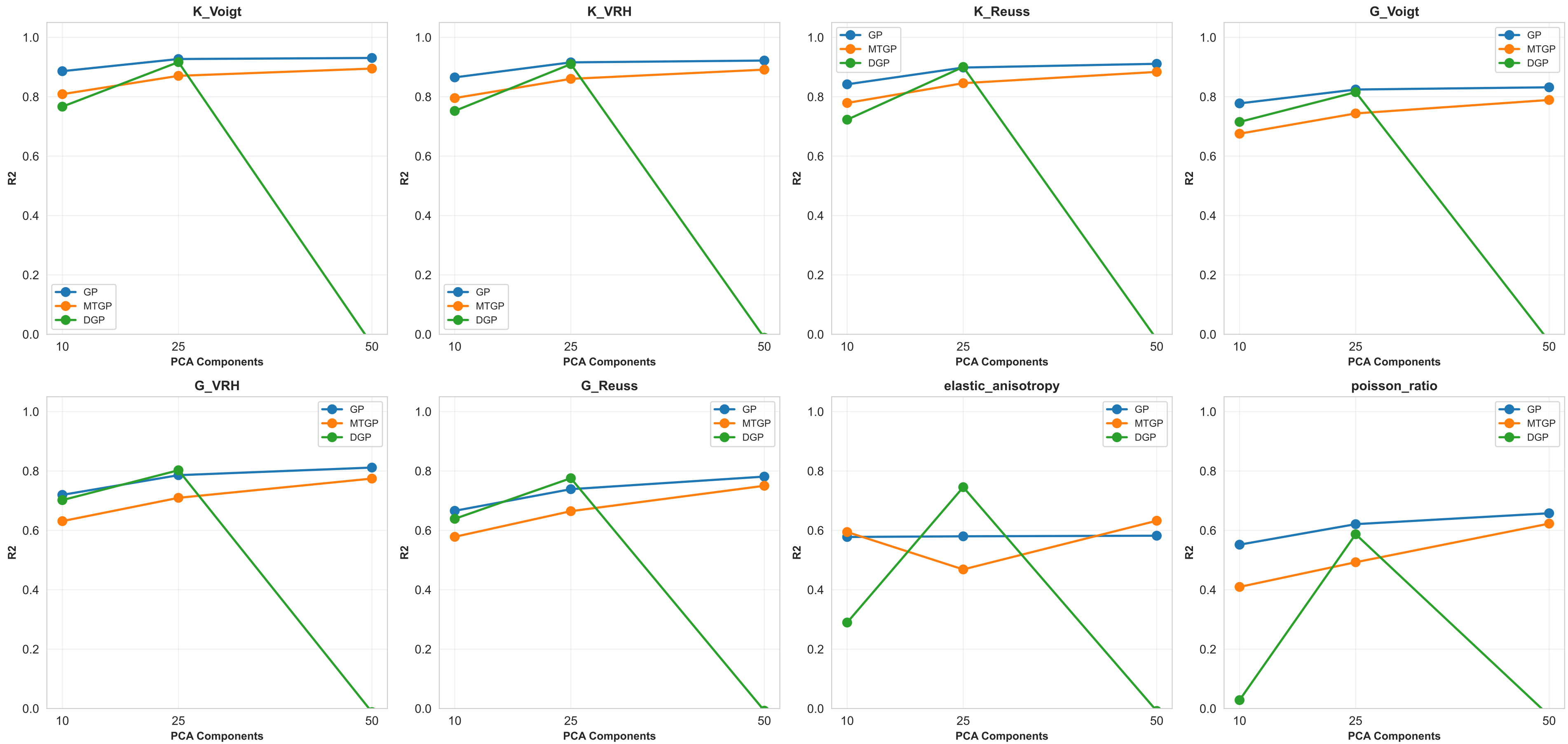
PCA Sensitivity Per Property: R2 (ORB Descriptor, n=500)
