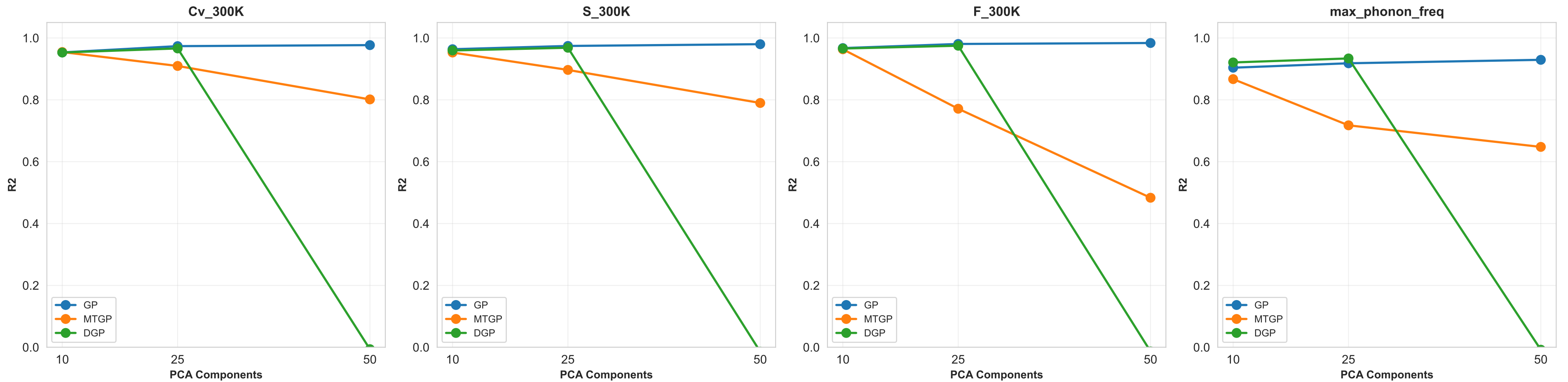
PCA Sensitivity Per Property: R2 (ORB Descriptor, n=500)
