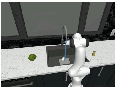
TurnOnSinkFaucet
