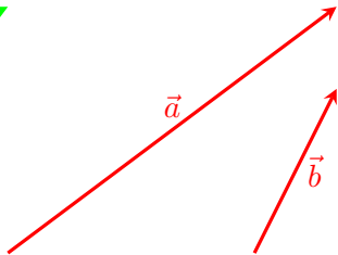
Nicht Kollineare Vektoren
