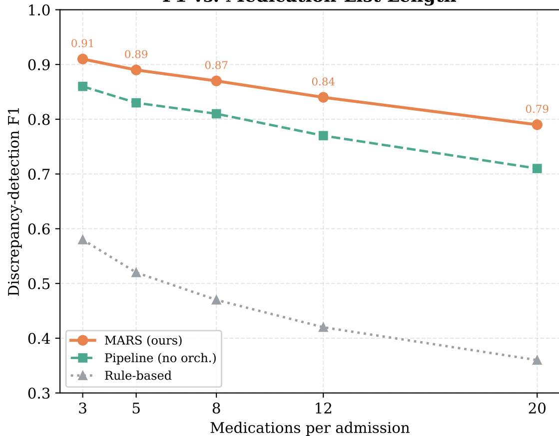
F1 vs. Medication-List Length
