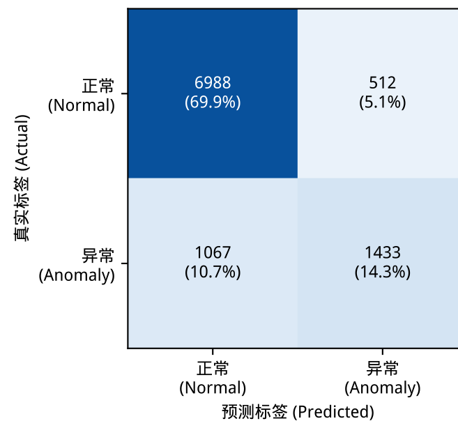
(f) PatchTST
