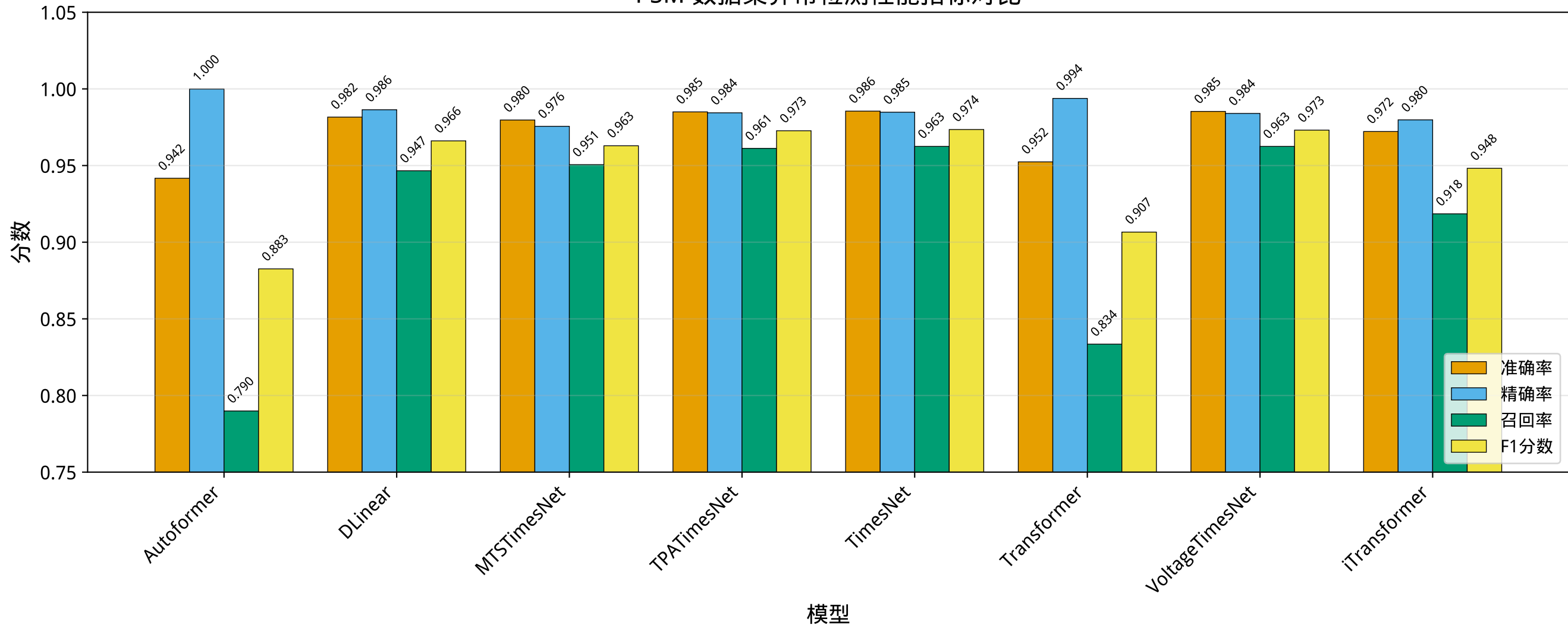
PSM 数据集异常检测性能指标对比
