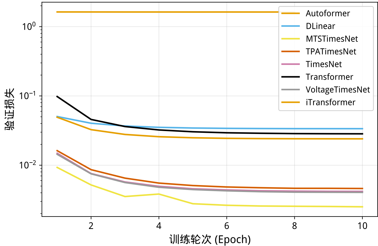
验证损失曲线对比
