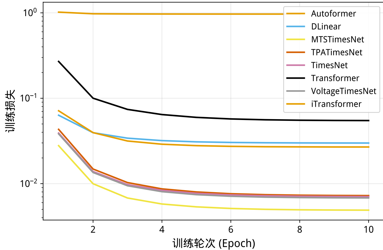
训练损失曲线对比
