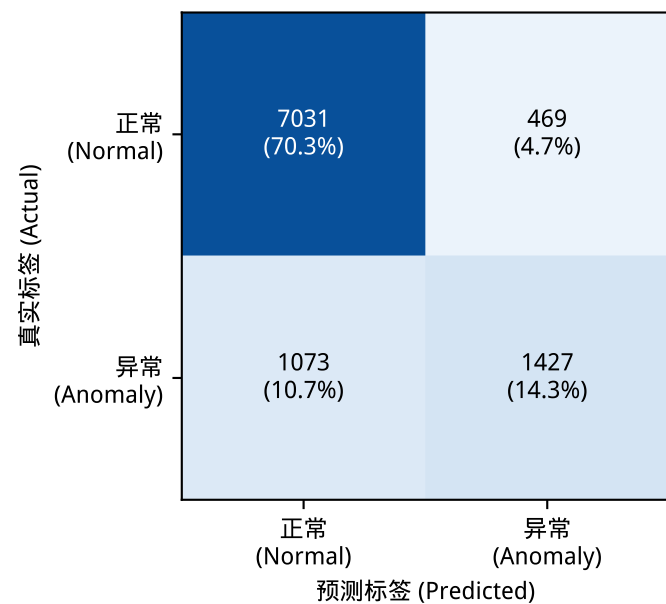
(d) TPA-TimesNet
