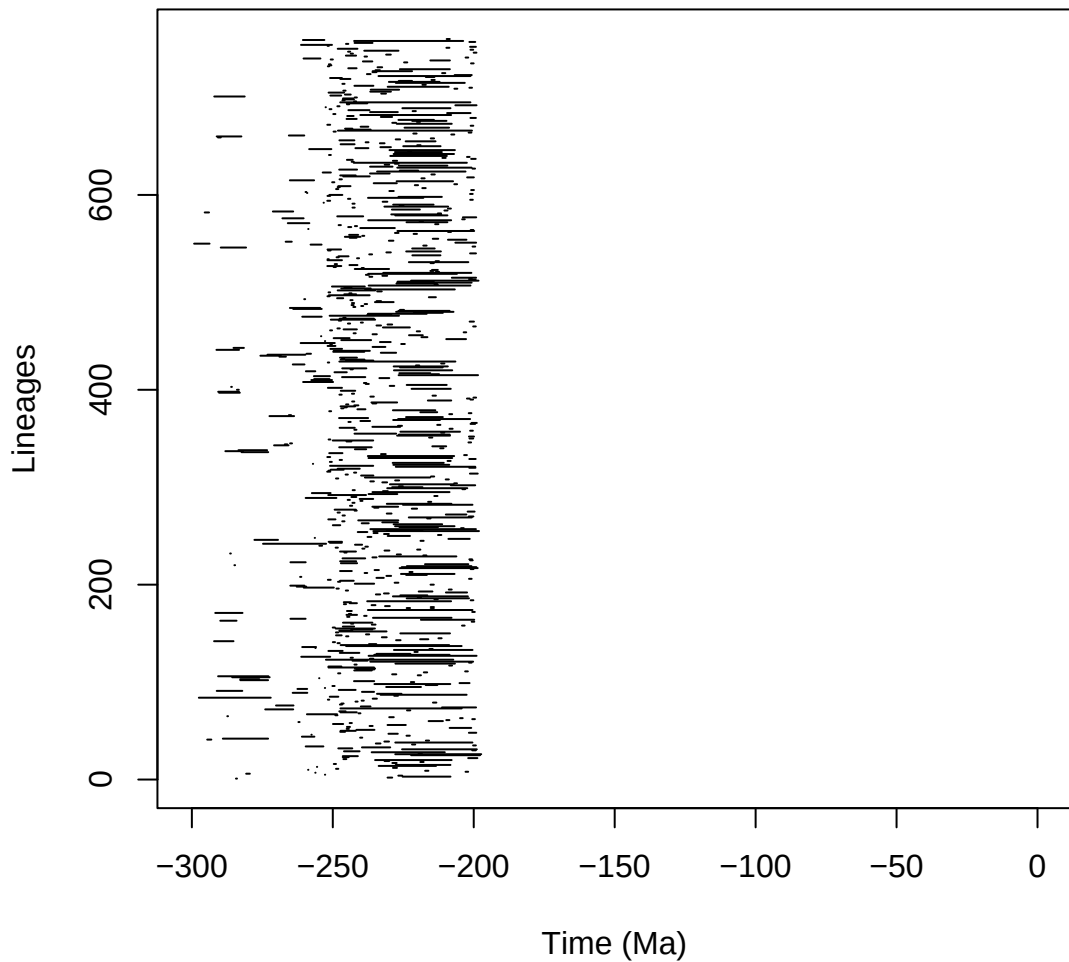
reptilia_pyrate_9_B_mcmc_G_COVhp_BD1-1_mcmc
