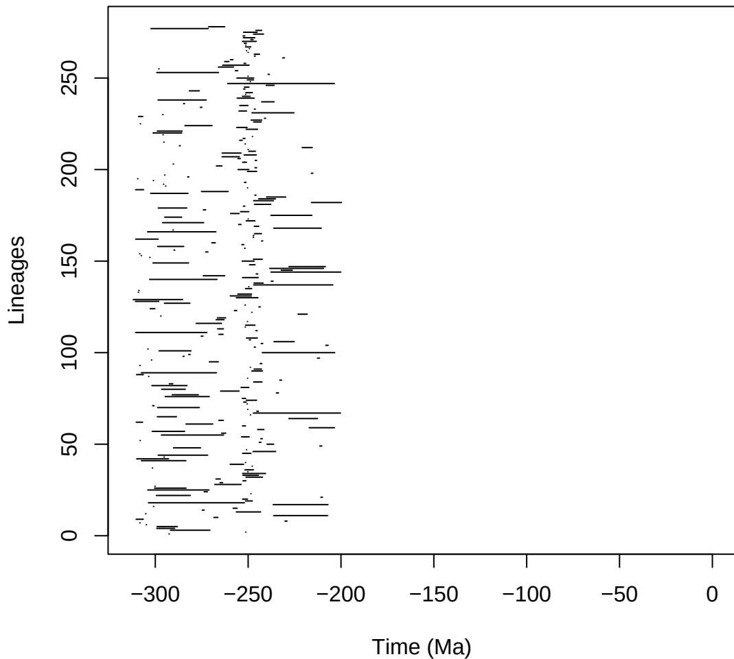
temnospondyli_pyrate_3_B_mcmc_G_COVhp_BD1-1_mcmc
