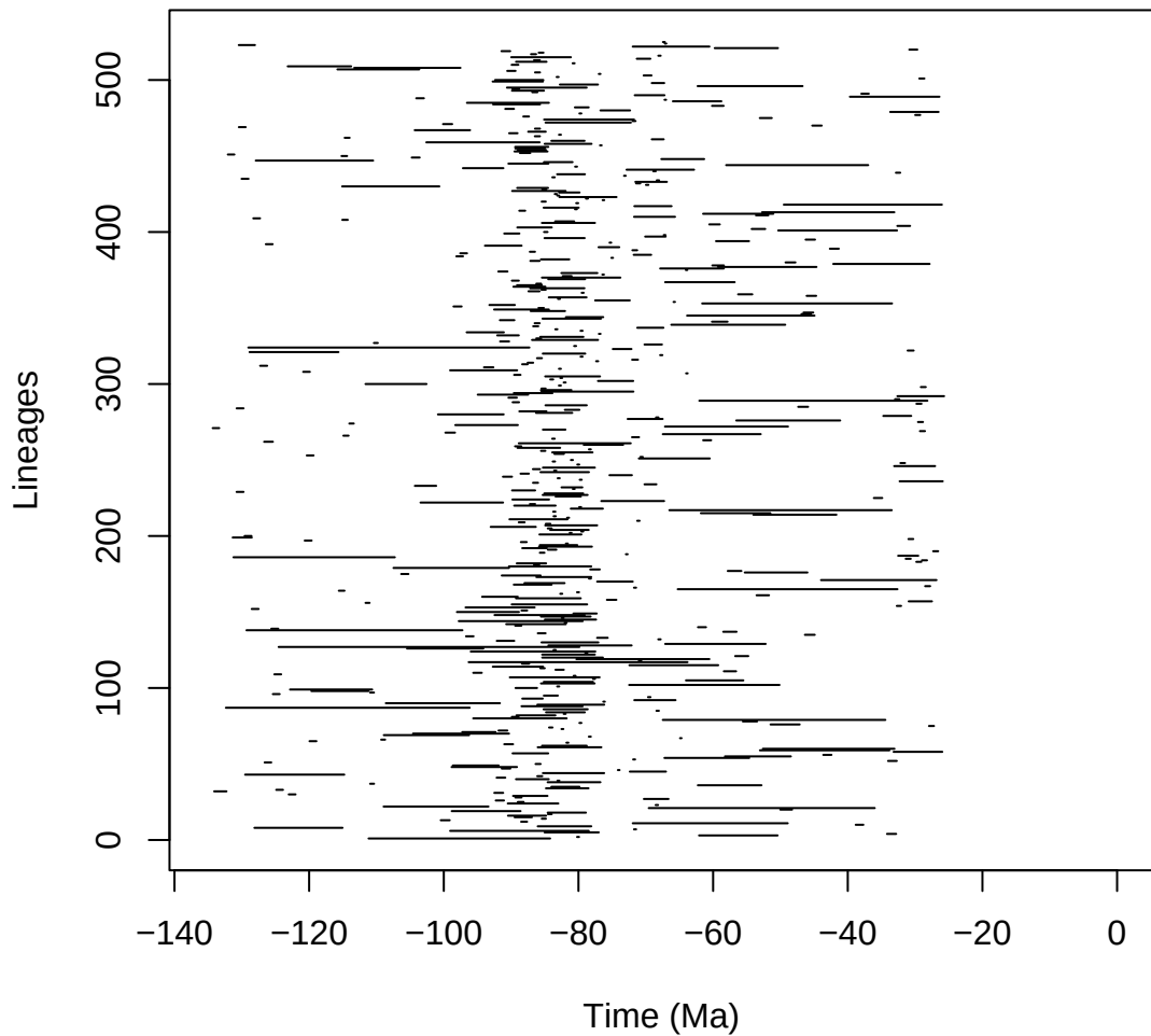
synapsida_pyrate_5_C_G_COVhp_BDS_mcmc
