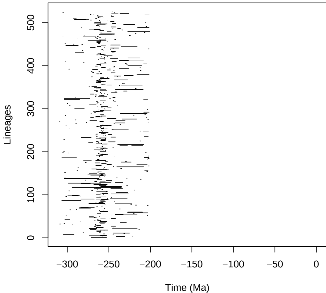
synapsida_pyrate_6_B_mcmc_G_COVhp_BD1-1_mcmc
