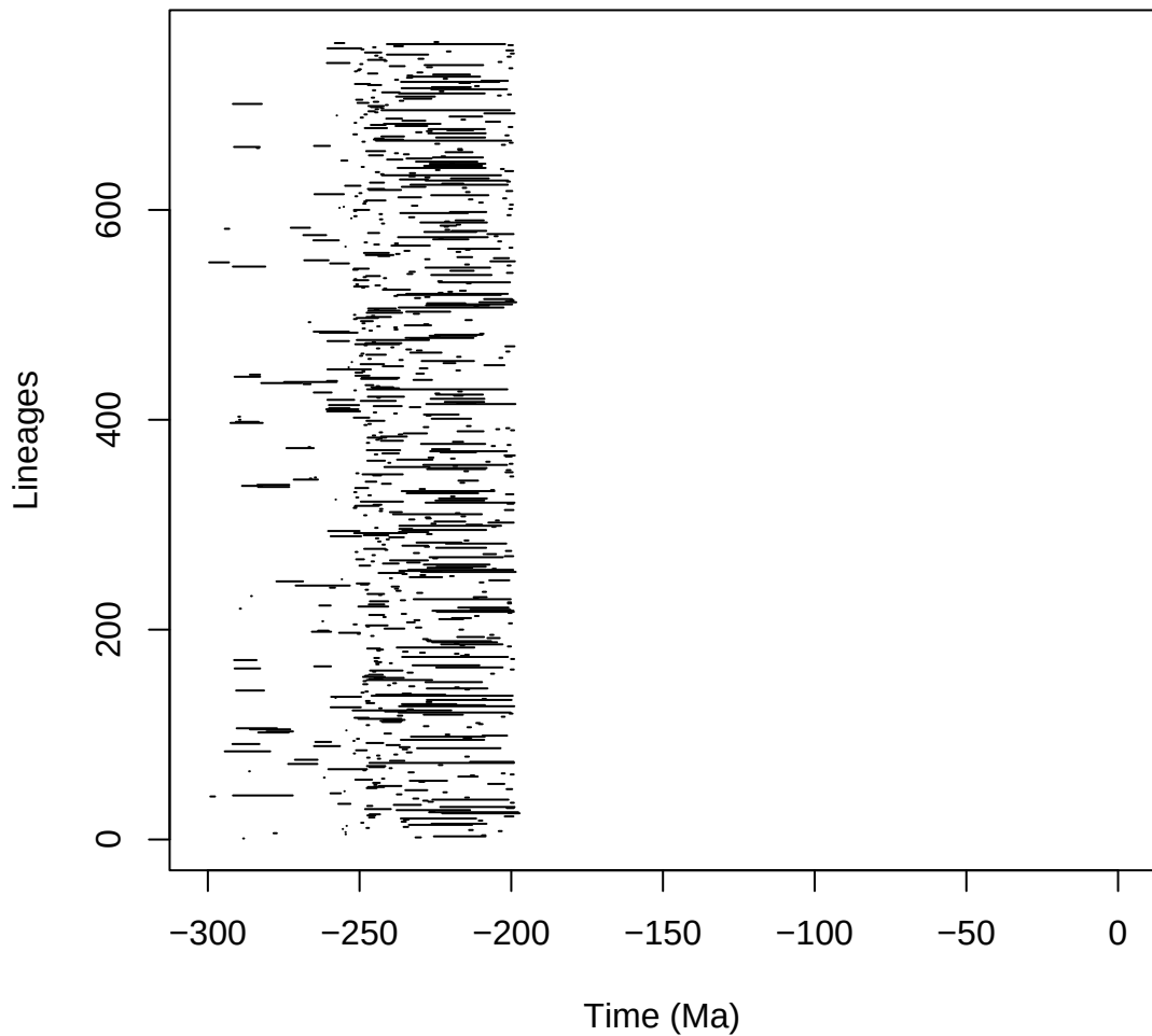
reptilia_pyrate_2_B_mcmc_G_COVhp_BD1-1_mcmc
