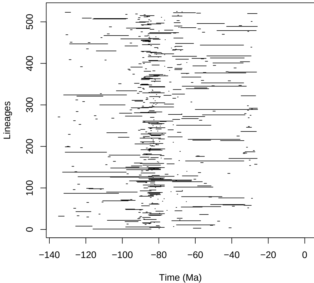
synapsida_pyrate_4_C_G_COVhp_BDS_mcmc
