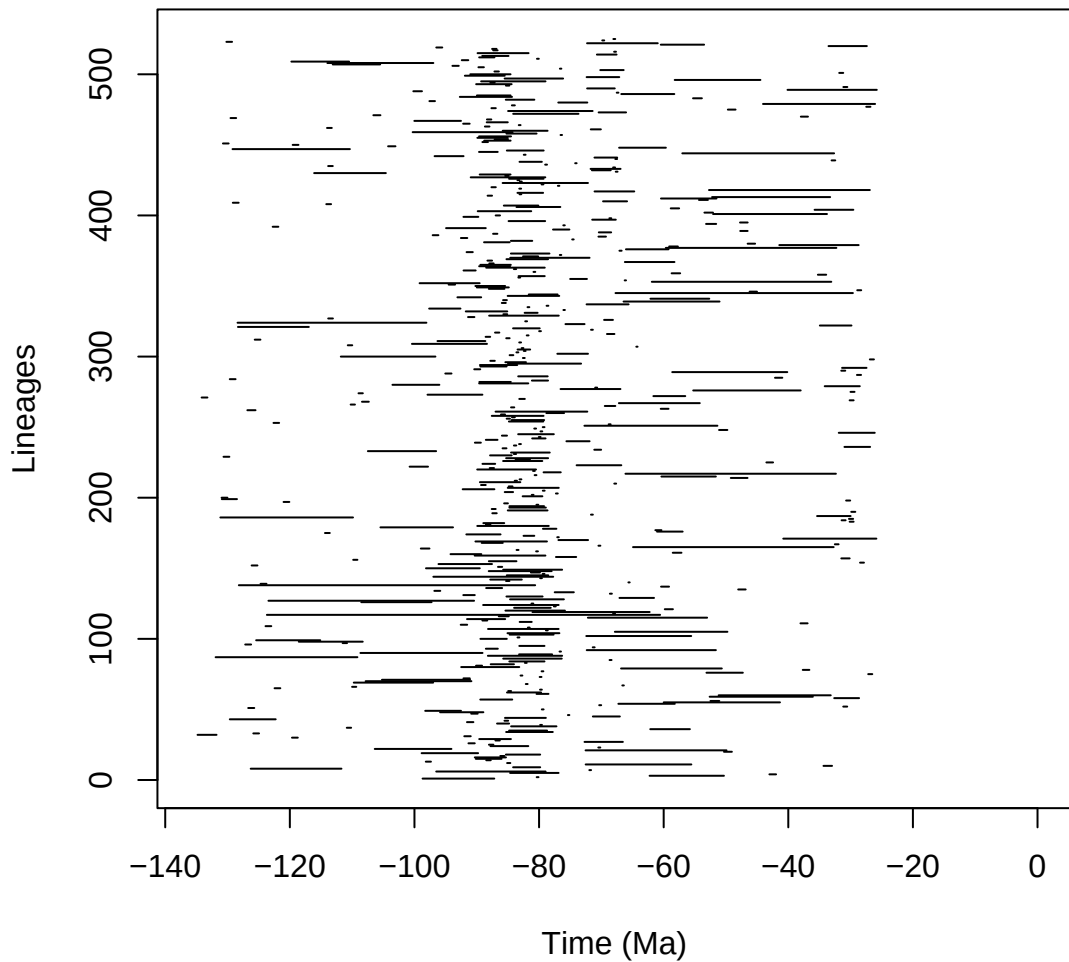
synapsida_pyrate_7_C_G_COVhp_BDS_mcmc
