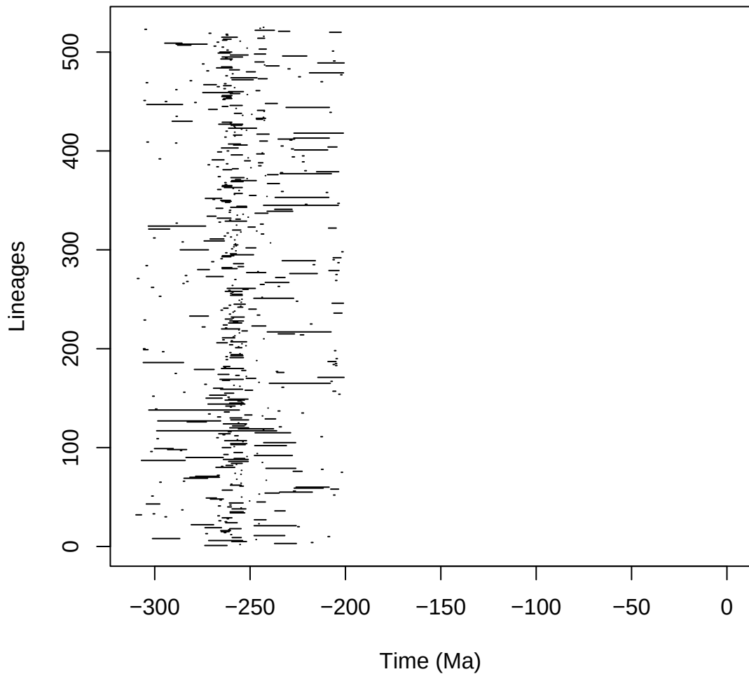
synapsida_pyrate_7_B_mcmc_G_COVhp_BD1-1_mcmc
