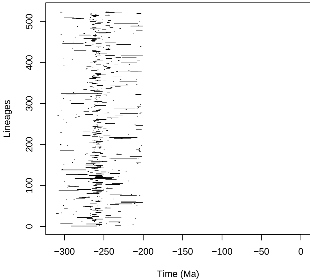
synapsida_pyrate_8_B_mcmc_G_COVhp_BD1-1_mcmc
