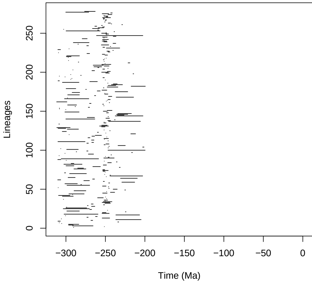
temnospondyli_pyrate_9_B_mcmc_G_COVhp_BD1-1_mcmc
