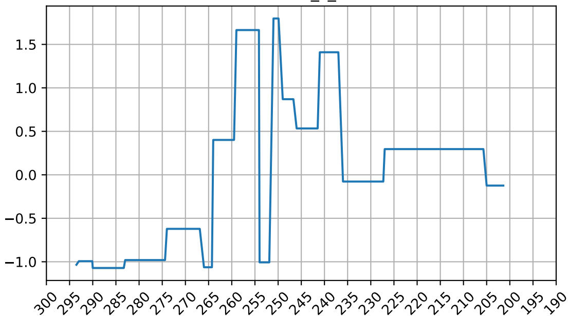
drymon_z_trans
