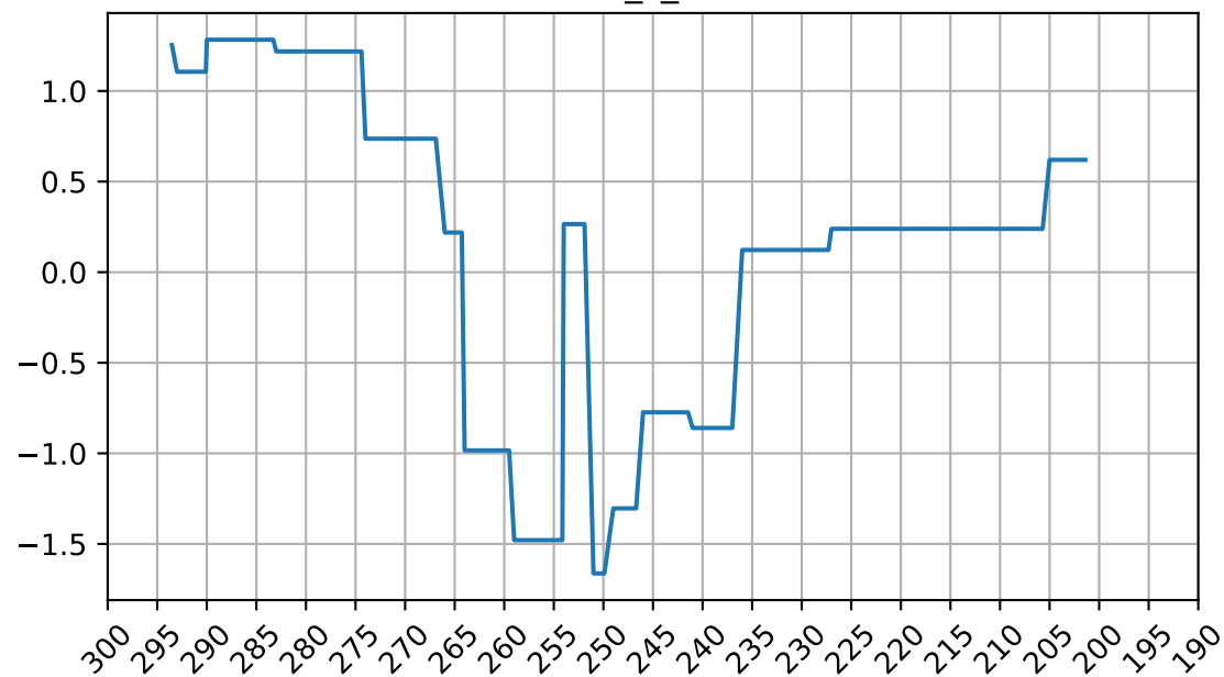
wetmon_z_trans
