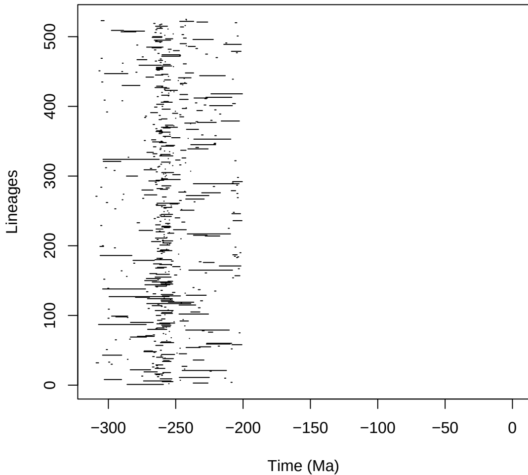
synapsida_pyrate_5_B_mcmc_G_COVhp_BD1-1_mcmc
