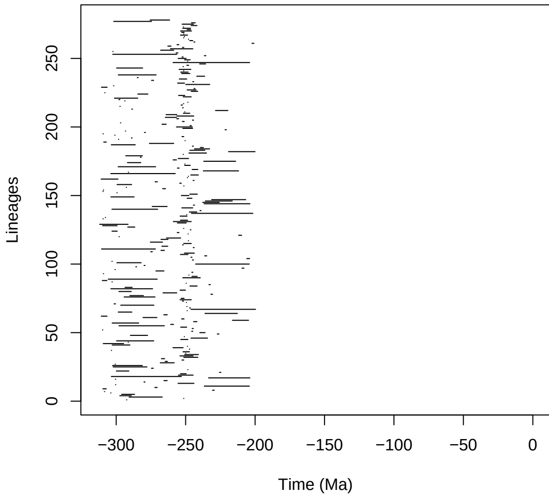
temnospondyli_pyrate_2_B_mcmc_G_COVhp_BD1-1_mcmc
