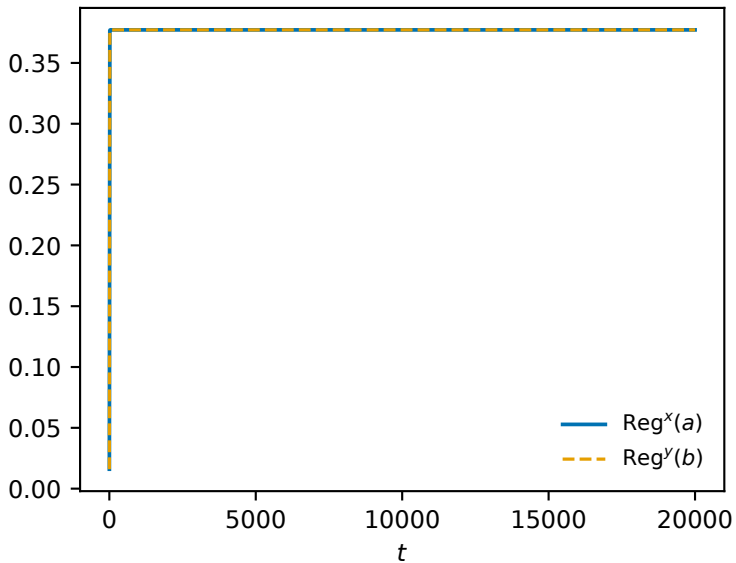
Hsieh OptDA self-play on G2
