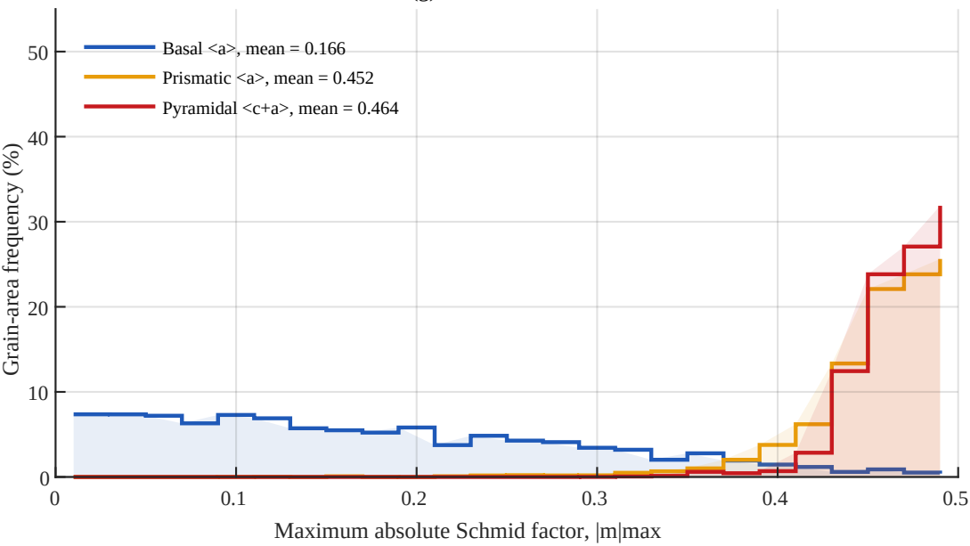
(g) 7d distribution
