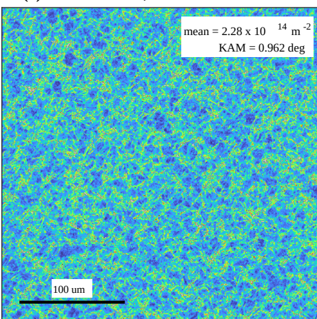
(d) 6.02d: 6.02 mm, 26.04% reduction
