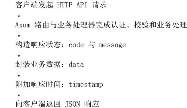
图 2 主要业务 API 的统一请求与响应流程 图 2 所示的统一响应结构适用于当前主要业务 API，不代表系统内所有接口均采用相同格式。页面和管理员接口需要携带有效 Token；管理员接口在身份验证后继续校验角色，避免普通用户访问用户管理、系统设置和审计数据。部分历史 API 仍使用参数查询或独立的响应结构。
