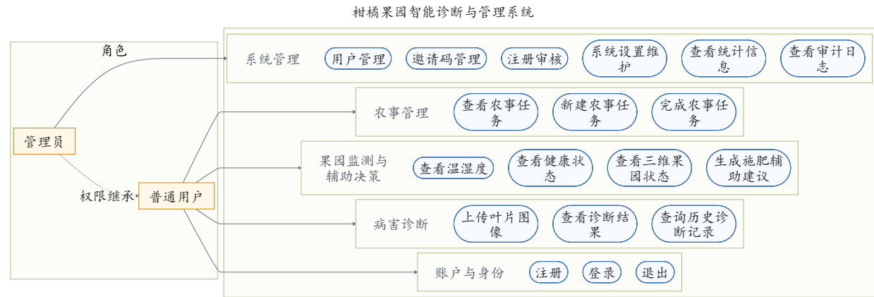
图 1 系统用例图
