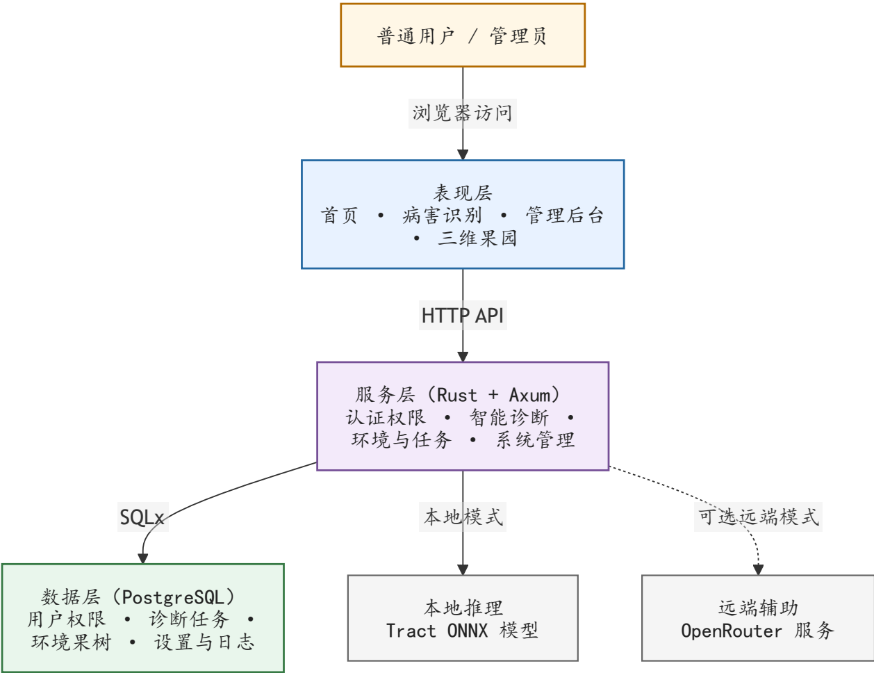
图 2 系统总体架构图 表 3 系统分层功能表
