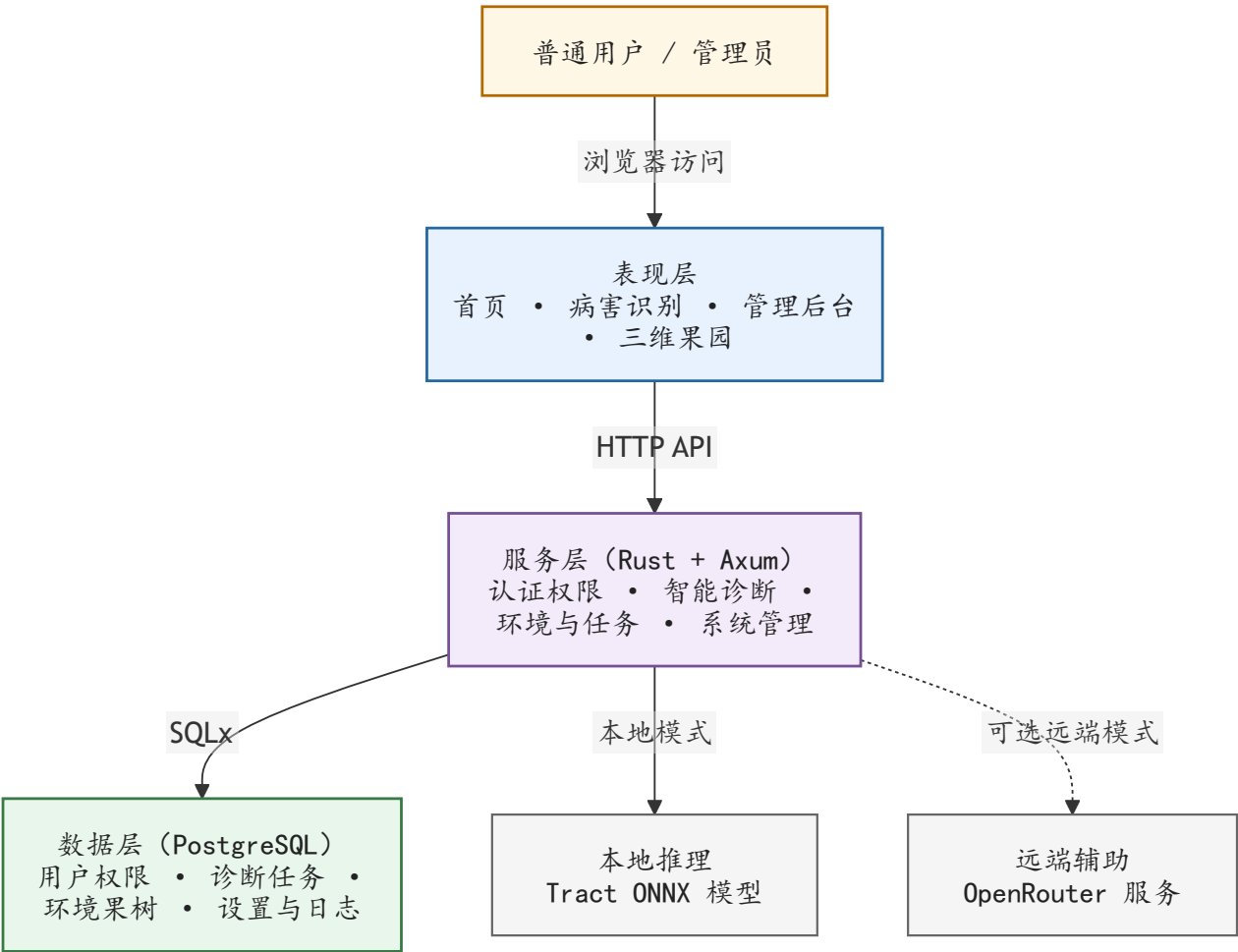
图 1 系统总体架构图
