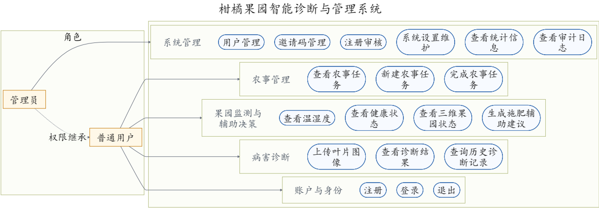
图 1 系统用例图
