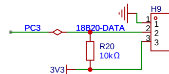
18B20插座
