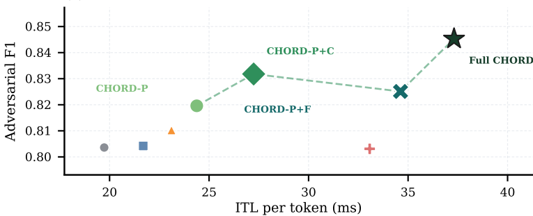
(a) LLaVA-v1.5-7B frontier
