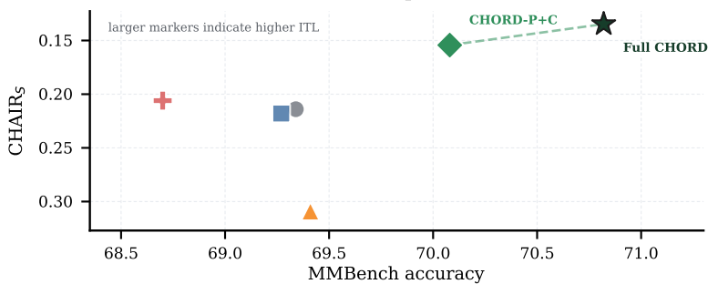
(d) InstructBLIP-7B trade-off map
