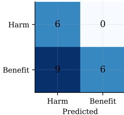
Virtual AdamW
