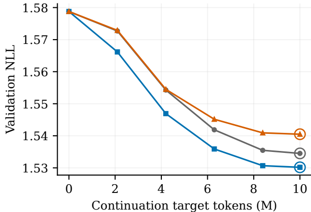
TinyStories
