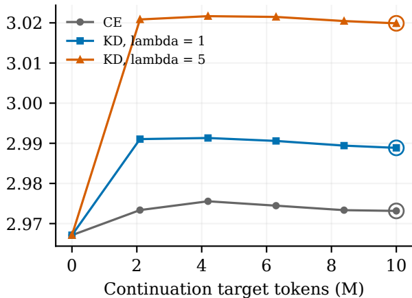
FineWeb-Edu
